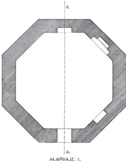
ALAPRAJZ. I.
