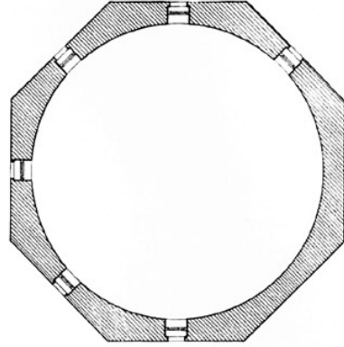
A KUPOLABOS ALAPRAJZ.
