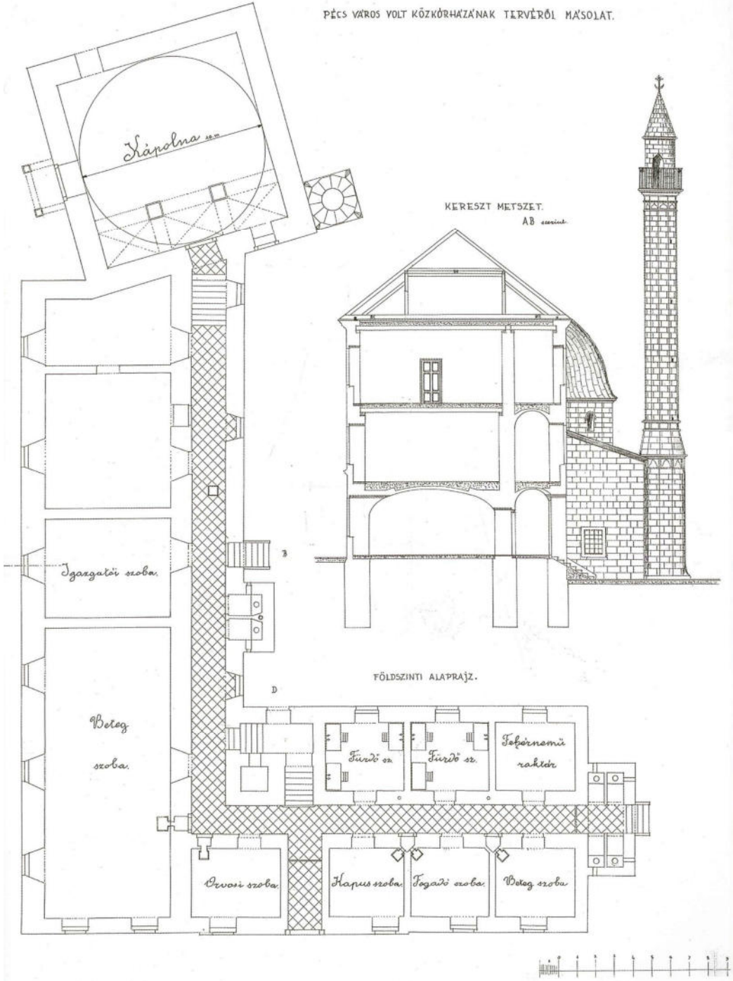
Yakovalı Hasan Paşa Câmii ile bitiřiğindeki hastanenin planı (1880, B. Sudâr'dan)
