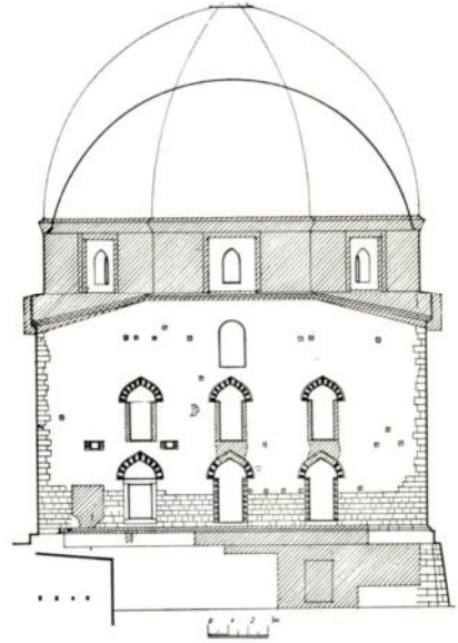
Gâzi Kâsım Paşa Câmii rölöve ve restitüsyonu (G. Gosztonyi 1941)
