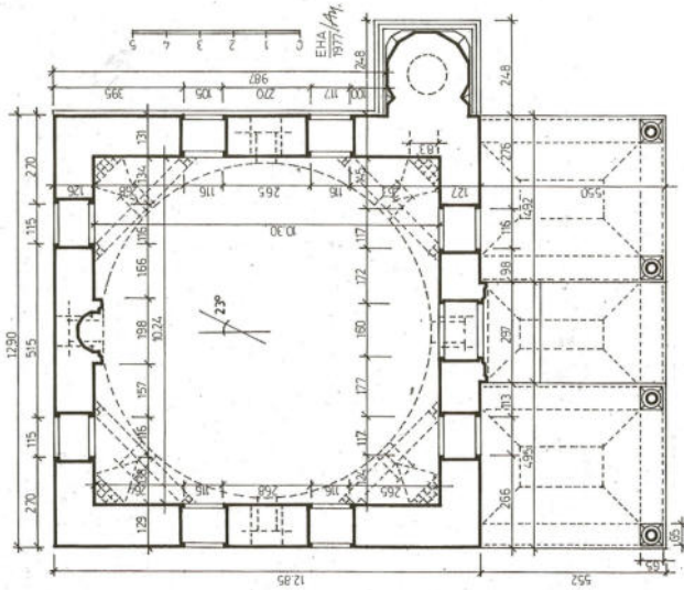
Yakovalı Hasan Paşa Câmii'nin restitüsyonu (E. H. Ayverdi)
