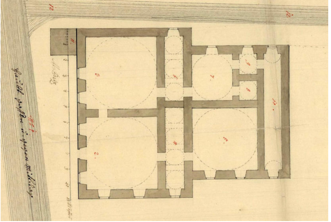
Ferhad Bey Hamamı'nın 1774 târihli plan ve cephe çizimleri
