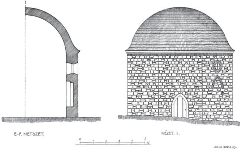
İdris Baba Türbesi'nin rölöve çizimleri (1917, F. Ernő'den, Çizim: János Sinogli)
