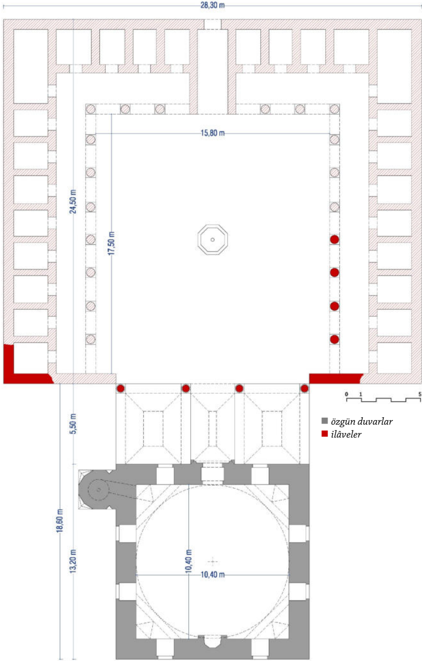
Yakovalı Hasan Paşa Câmii ve Mevlevihâne'nin restitüsyon önerisi Tekkenin bulunduğu alanda yapılan kazı sonrası çıkan izlere ait çizim müzede sergilenmektedir. Bu plan, müzede levhadan işlenerek yeniden çizilmiştir. Bkz. Mevlevihâne
