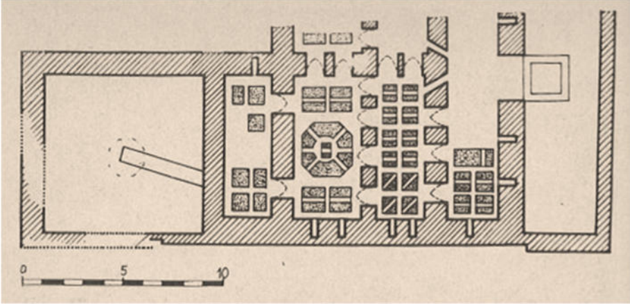
Memi Paşa Hamamı'nın cehennemlik seviyesi planı (Gerö 1987'den)
