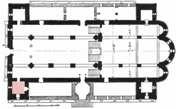
Peçuy Katedrali'nin planı (Gerecze 1893'ten) Kitâbe, renkli gösterilen kulededir.
