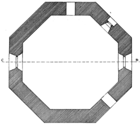
ALAPRAJZ. II.
