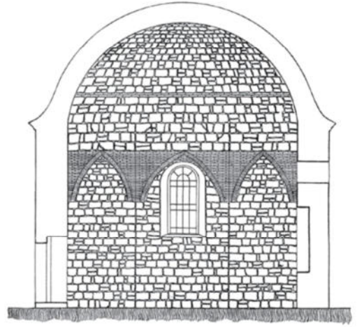
A-B METSZET.
