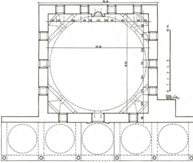
Ekrem Hakkı Ayverdi'nin restitüsyon önerisi, 1976 (Çizim: İ. Aydın Yüksel)
