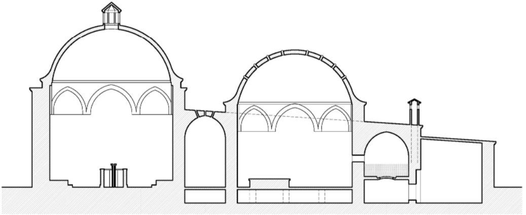
Memi Paşa Hamamı restitüsyon denemesi (MEY, 2024)
